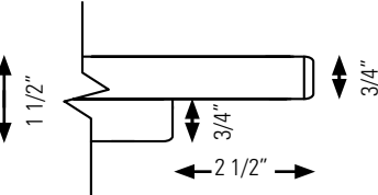
Edge Detail - Casegoods
